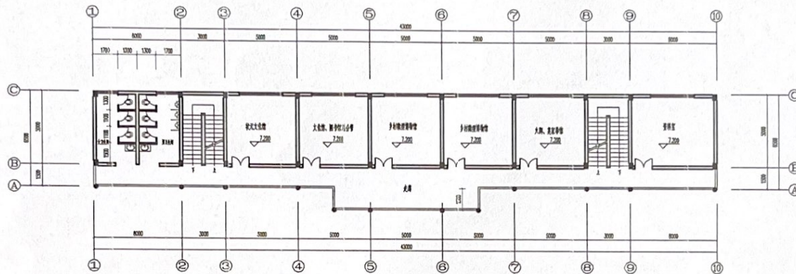
三层平面图 1:100 本层建筑面积: 279.5m 2
