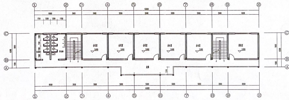
二层平面图 1:100 本层建筑面积: 279.5m 2
